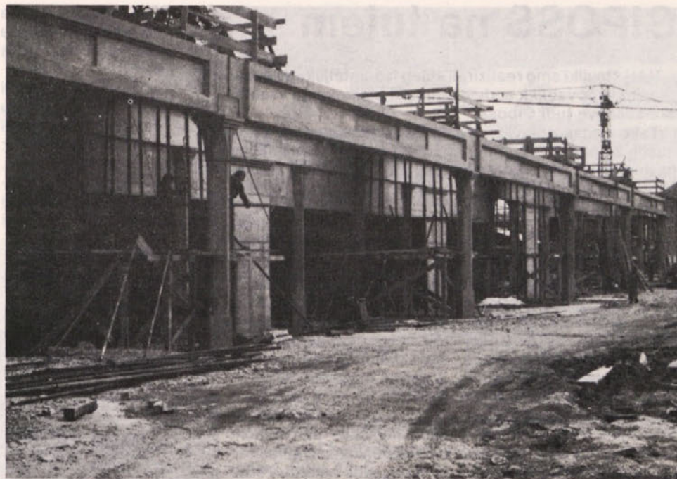
V Rogaški Slatini je v gradnji nov poslovni center. Posebej oblikovane montažne elemente so z novimi opaži izdelali v tozd IGM, obrat Rogaška Slatina. Foto Vili Š.
