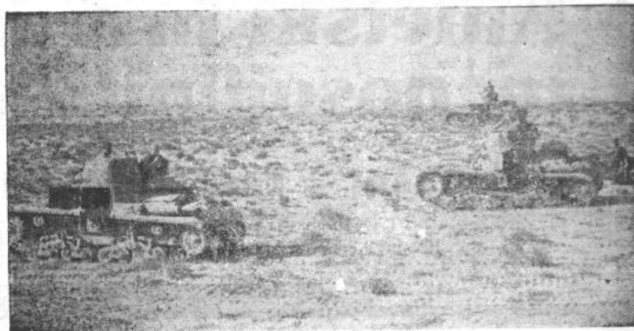
Italijanski tanki pri prodiranju skozi afriške puščave
