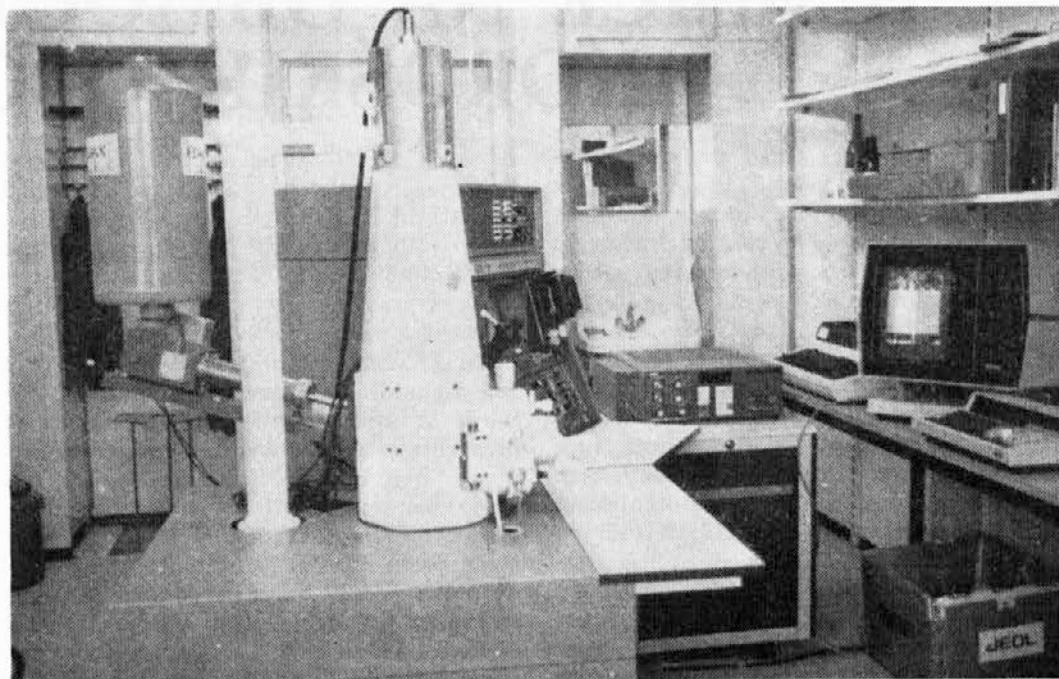
Raster elektronski mikroskop v Železarni Ravne
