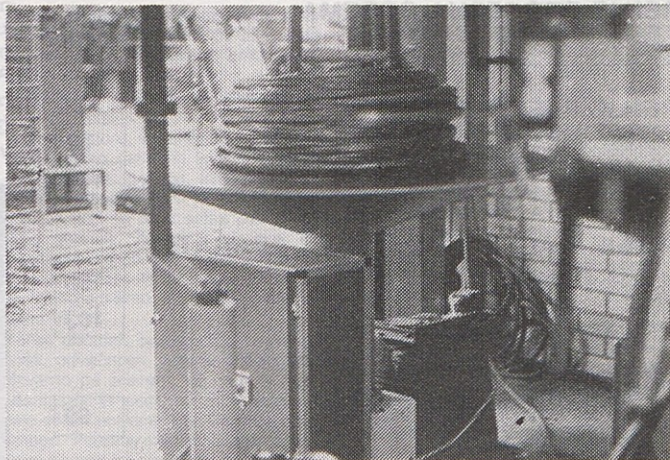
Računalniško vodeni stroj za izdelavo žičnih elementov so izpopolnili z odvijalno napravo, ki so jo izdelali v Gorenju Procesna oprema
