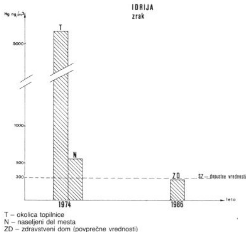
Sl. 1: Koncentracije hlapov živega srebra v zraku naseljenega dela mesta Idrija v času polne proizvodnje (1974) in pri zmanjšani proizvodnji živega srebra v rudniku ter dopustne vrednosti, ki jih uporabljajo v Sovjetski zvezi.
