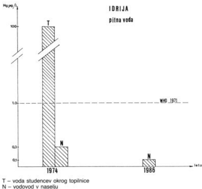
Sl. 2: Koncentracije živega srebra v pitni vodi v Idriji v času polne proizvodnje (1974) in pri zmanjšanju proizvodnje (1986) živega srebra v rudniku ter priporočene dopustne vrednosti elementarnega živega srebra v pitni vodi (WHO 1971).
