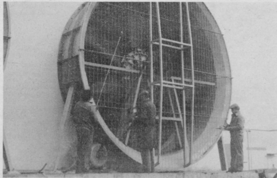
Preizkus aksialnega ventilatorja, premera 6 metrov.
