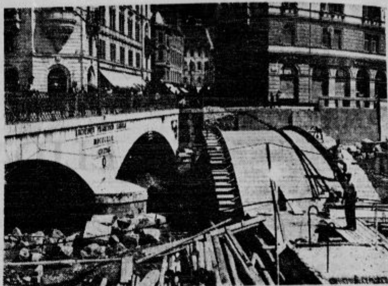
Franciskanski most v Ljubljani bo dobil dva nova tovariša: enega na desni, enega na levi. Sam ne zmore več vedno večjega prometa. Ogradje za novi betonski most na zgornji strani so že postavili. Pravijo, da bo tromostovje zelo lepo in nad pokrugi milijon dinarjev bo stalo.
