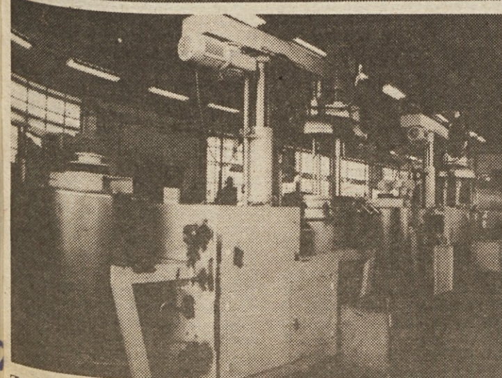
Zgoraj: Bobnasti filter, spodaj aparat za vakumsko kuhanje, mešanje in dodelavo medu.
