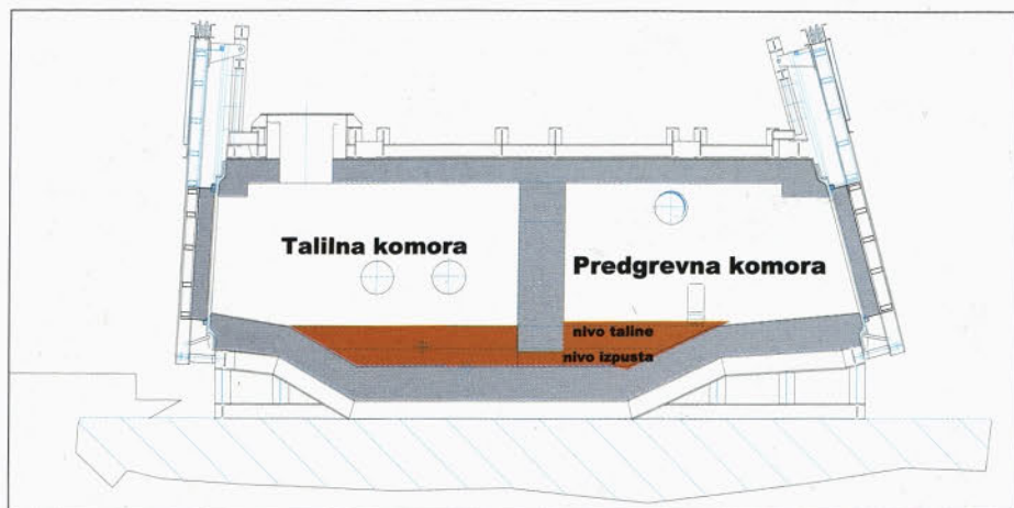
Slika 1: prerez dvokomorne peči
