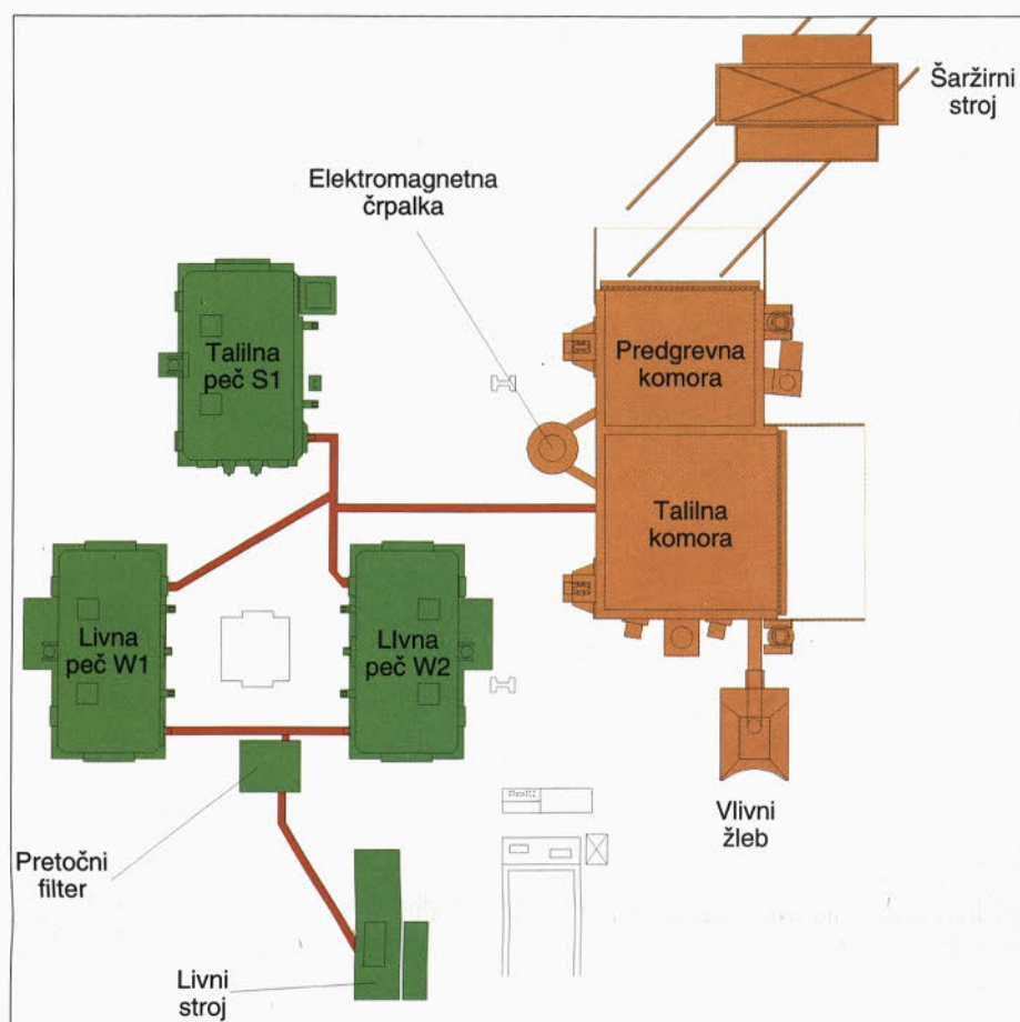
Slika 2: Nova talilna peč R1
