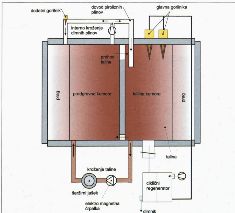
Slika 3: Shematski prikaz delovanja peči
