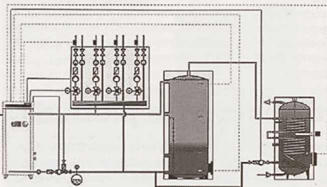
Hidravlična shema sodobnega kotla na lesno biomaso
