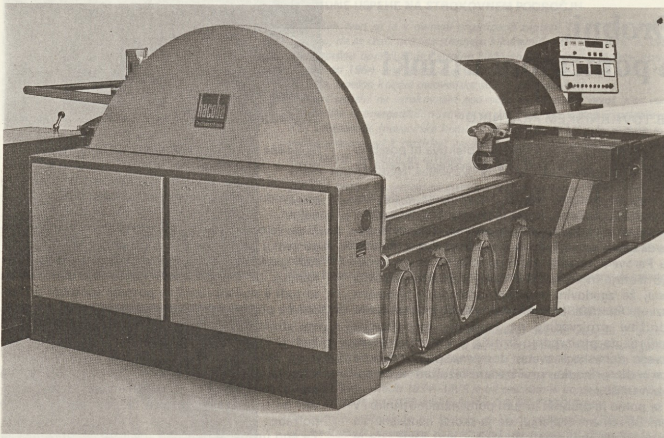
Moderno saško snovalo z elektronskim vodenjem
