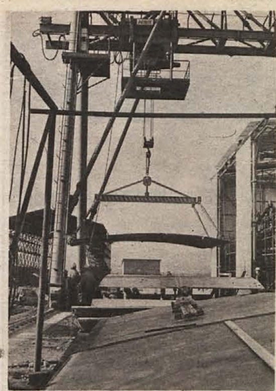
Pri graditvi jedrske elektrarne v Krškem sodelujejo slovenska in hrvaška podjetja. Trenutno delajo tam delavci našega Gradisa in Hidroelektrne iz Zagreba, montažo pa bosta prevzela hrvaško podjetje „Djuro Djaković“ in Hidroelektra iz Maribora. (Foto: J. Teppey)
