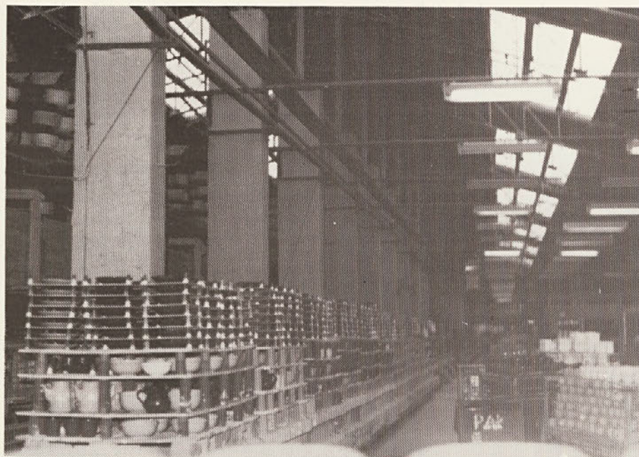
Drugo glazirno žganje v tunelski peči pri temperaturi 1040°
