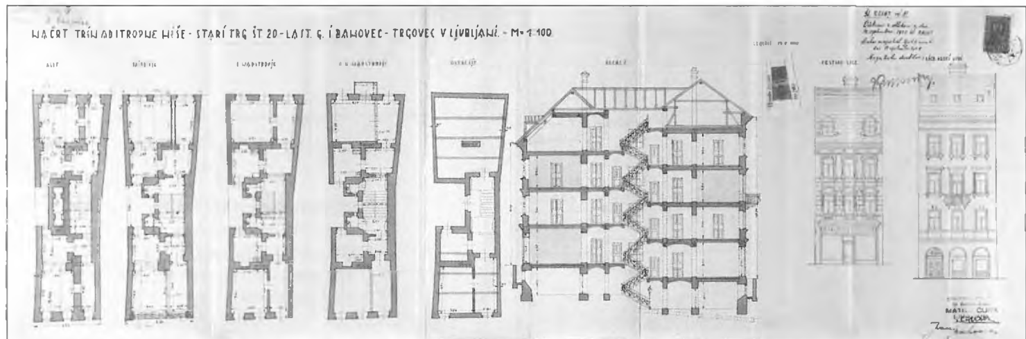
15 Stanovanjska hiša na Starem trgu 20, 1928, tlorisi etaž, prerez, fasadi in situacija, adaptacija; kolorirana kopija / 101,7 x 33,7, ZAL, Mesto Ljubljana, gradbena registratura (LJU 493), Reg IV, f. 640
