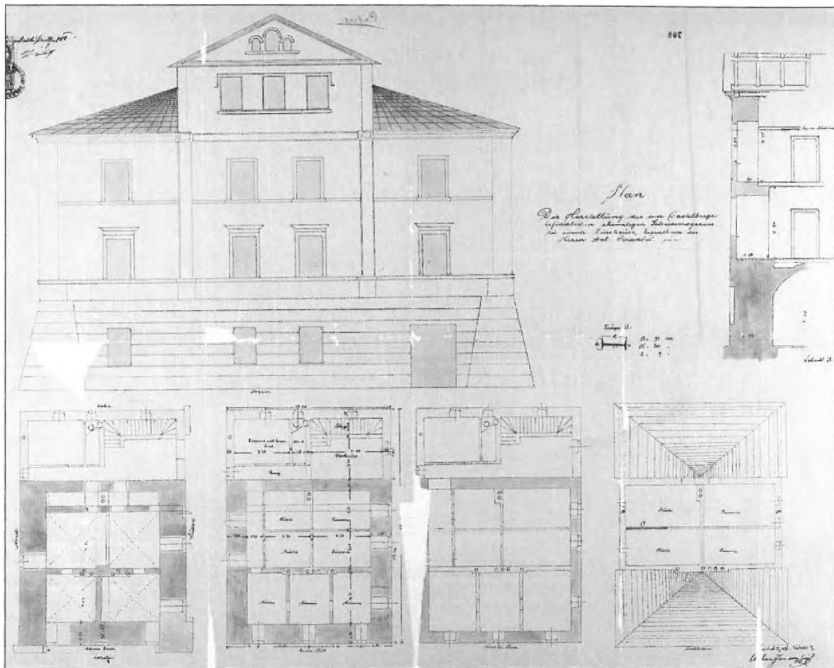
19 Kubelka, Stanovanjska hiša na Osojni poti 3, 1876, fasada, prerez in tlorisi etaž, gradnja; kolorirana matrica / 74,4 x 53,8, ZAL, Načrti (LJU 334), Restavrirani in konservirani načrti, mapa 8, 18 (fol. 708)
