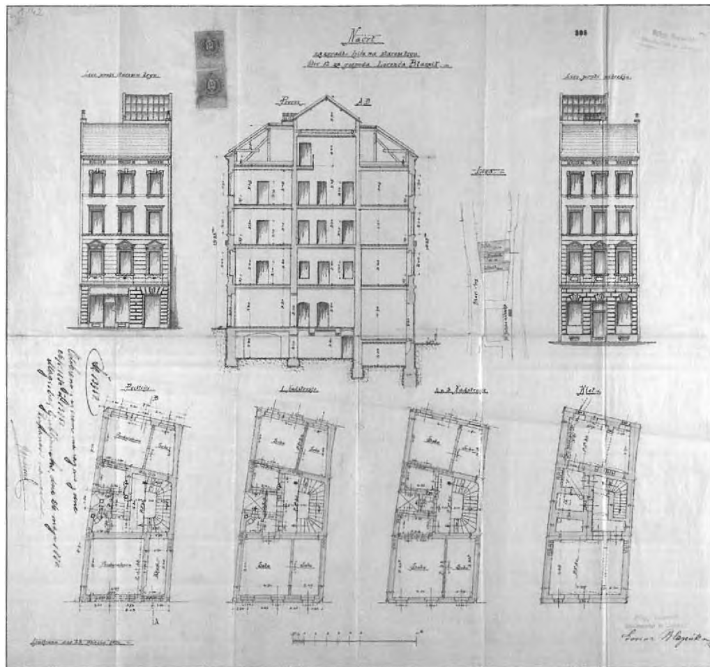
14 Stanovanjsko-trgovska hiša na Starem trgu 12, 1896, fasadi, prerez, tlorisi etaž in situacija, nadgradnja; kolorirana matrica / 63,6 x 59, ZAL, Mesto Ljubljana, splošna mestna registratura (LJU 489), Reg I, f. 1142, fol. 398
