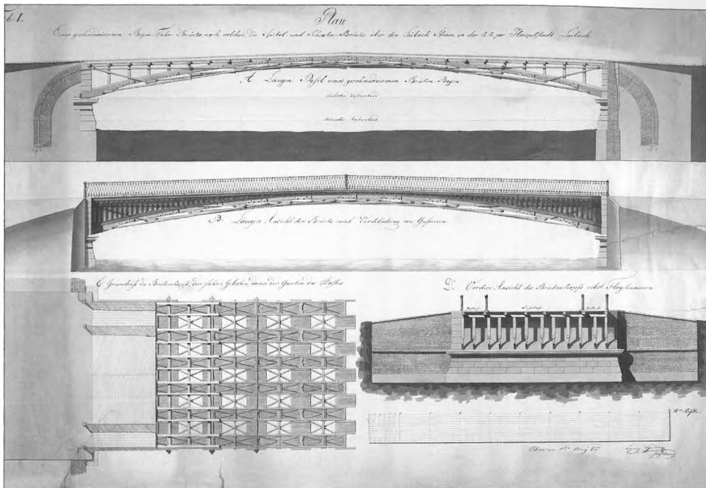
11 Franz Hutter, Čevljarski most, obočni most iz gibkega železa, 1837, vzdolžni prerez, pogled, tloris-prerez in prečni prerez, neizvedeni projekt; kolorirana matrica / 96,9 x 63,8, ZAL, Načrti (LJU 334), mapa 01/1, 1
