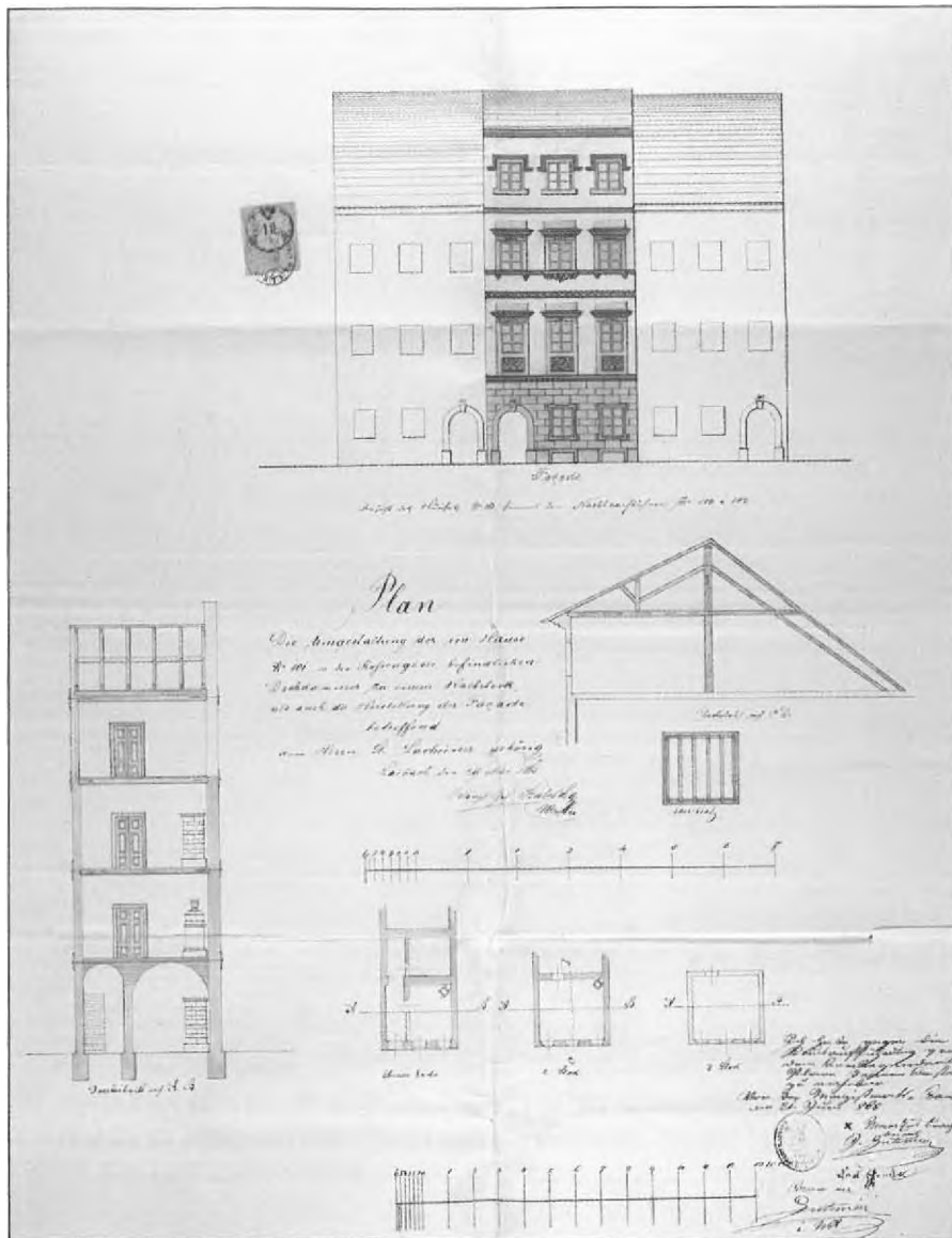
20 Kubelka, Stanovanjska hiša v Rožni ulici 7, 1865, fasada, prereza in delni tlorisi etaž; kolorirana matrica / 48,9 x 63, ZAL, Mesto Ljubljana, splošna mestna registratura (LJU 489), Reg I, f. 753, fol. 316
