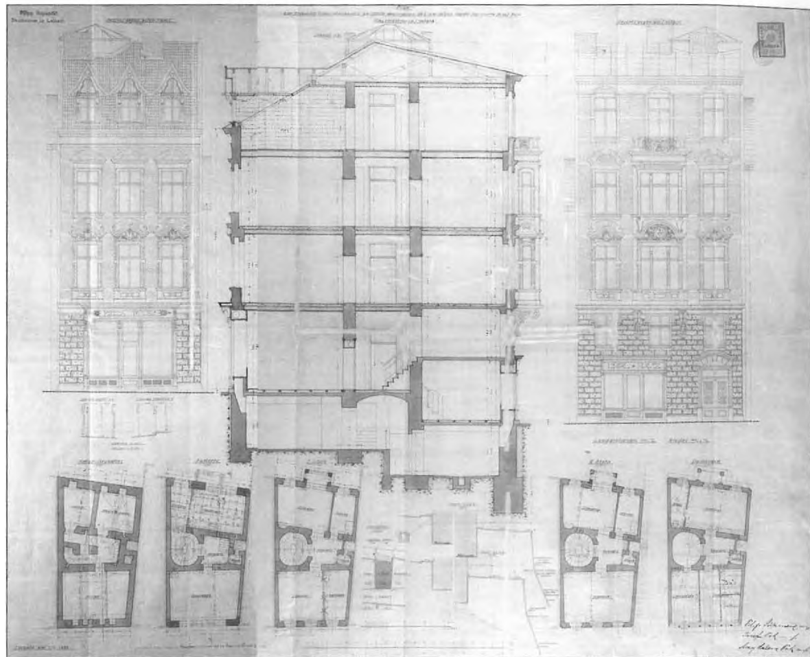
13 Stanovanjsko-trgovska hiša na Starem trgu 8, 1898 , fasadi, prezez in tlorisi etaž, adaptacija; kolorirana kopija / 82,8 x 67,9, ZAL, Načrti (LJU 334), Restavrirani in konservirani načrti, mapa 1, 22 (fol. 579)
