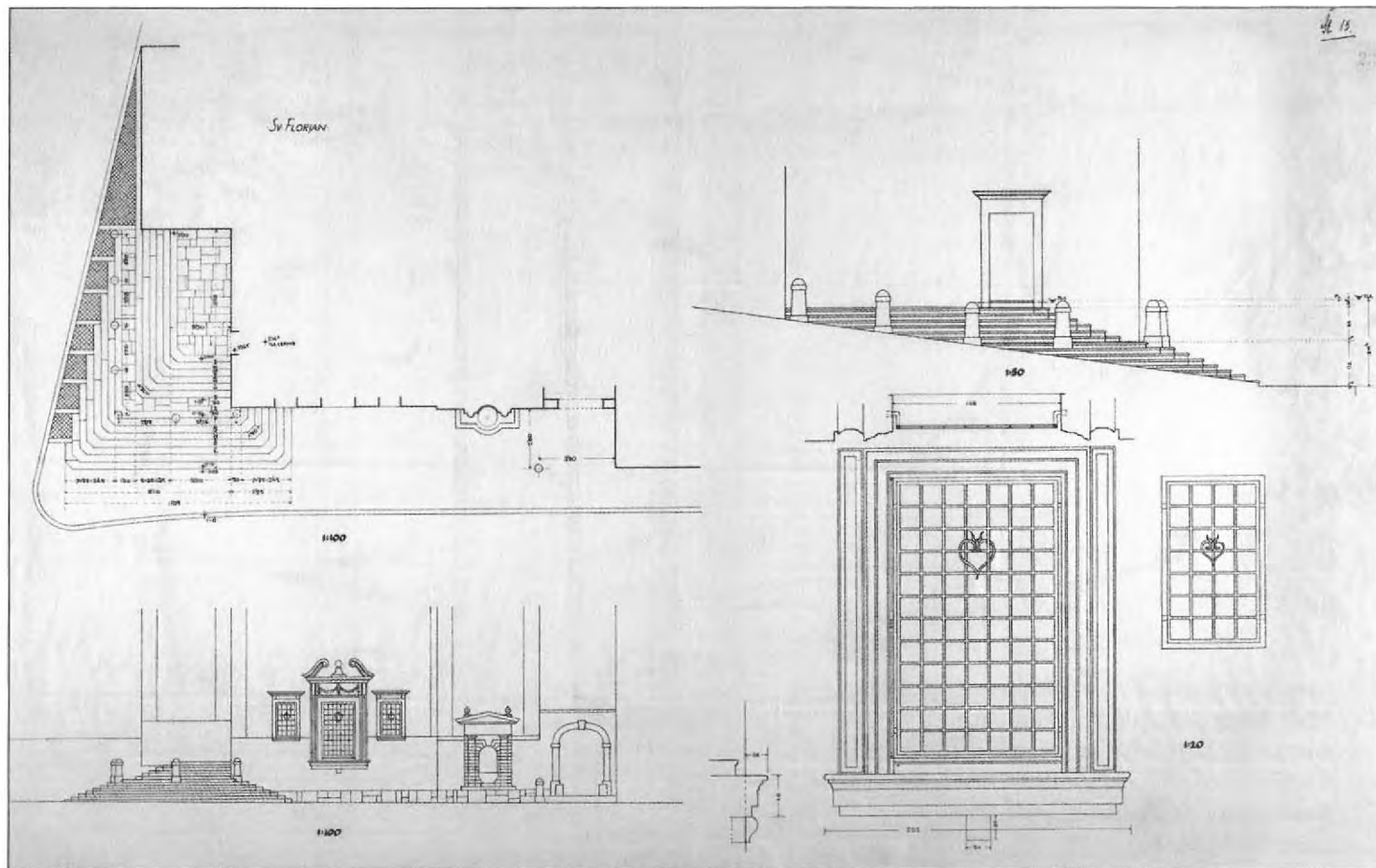
18 Stopnišče in okno cerkve sv. Florijana na Gornjem trgu/Ulici na Grad, 1932/1933, tloris in pogled stopnišča, del fasade na Gornjem trgu, pogled, tloris in profil okna, prerez okenskega okvira, gradnja stopnic in adaptacije; matrica / 75,2 x 42,5, ZAL, Načrti (LJU 334), mapa 13/3, 9 (fol. 23)
