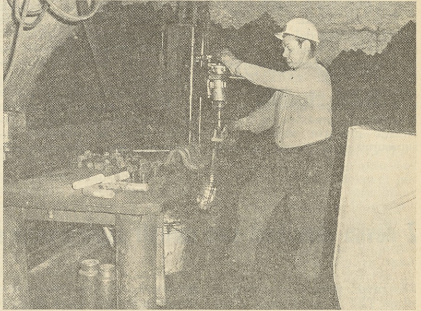
Franc Medvešek kompletira objemke za TH podporje v jami Hrastnik, IV. obzorje. (Foto A. Bregant)
