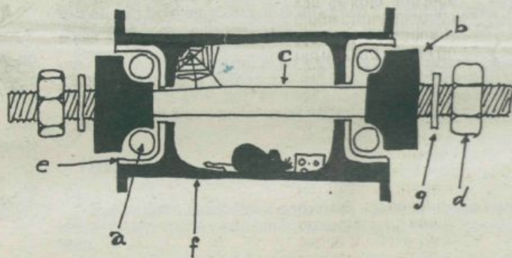
Slika 2. Pesto v prerezu: a - kroglice, b - konus, c - os, d - protimatica, e - čašica, f - pesto, g - zobaba podložitka.
