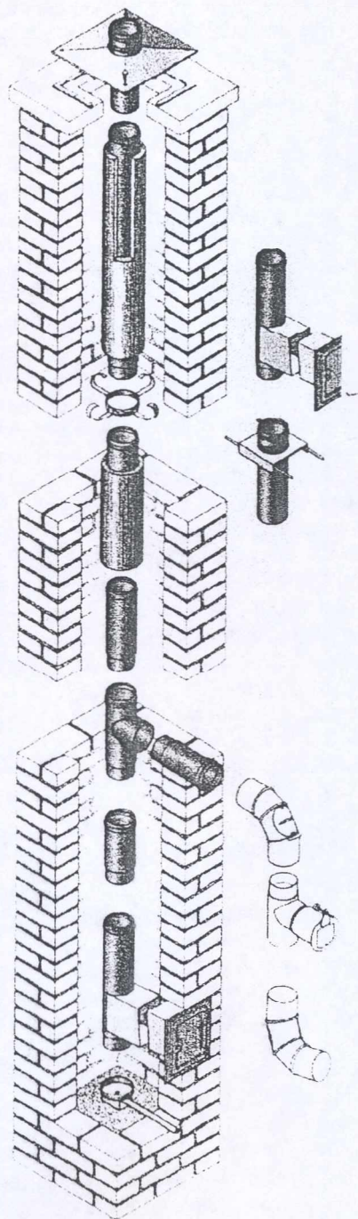
Shema dimnika
