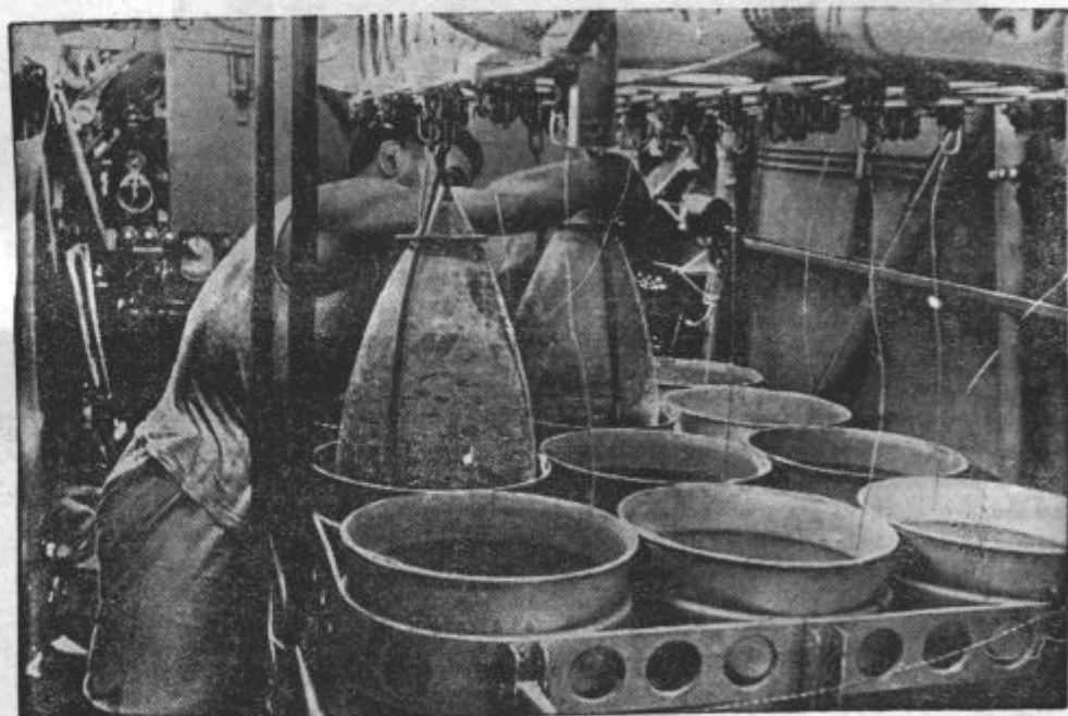
BOMBNI PROSTOR V LETALU. Pogled v prostor za bombe v italijanskem letalu
