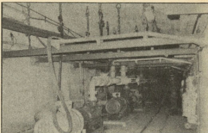
Novo vodno črpališče na koti +30 v jami Škale
