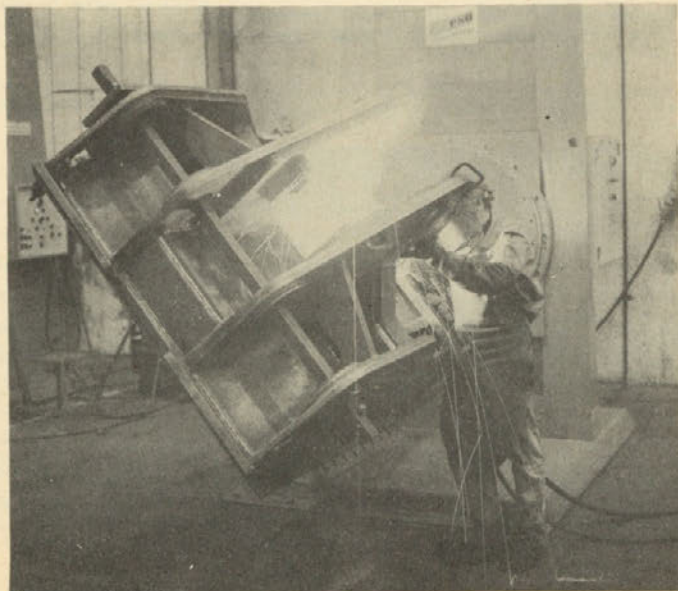
PTO-45, pozicioner za težke obdelovance
