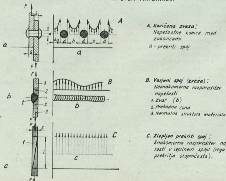
PRIMERJAVA RAZPOREDITVE NAPETOSTI PRI RAZLIČNIH VEZAVAH DVEH MATERIALOV
