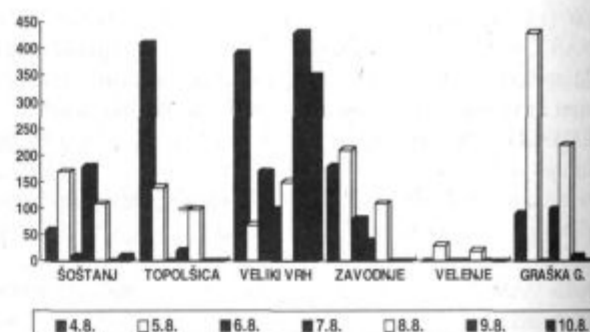
MAKSIMALNE POLURNE KONCENTRACIJE SO 2 od 4. avgusta do 10. avgusta 1997
