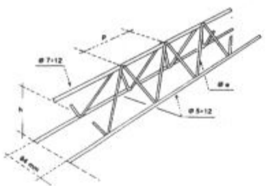
REŠETKASTA ARMATURA
