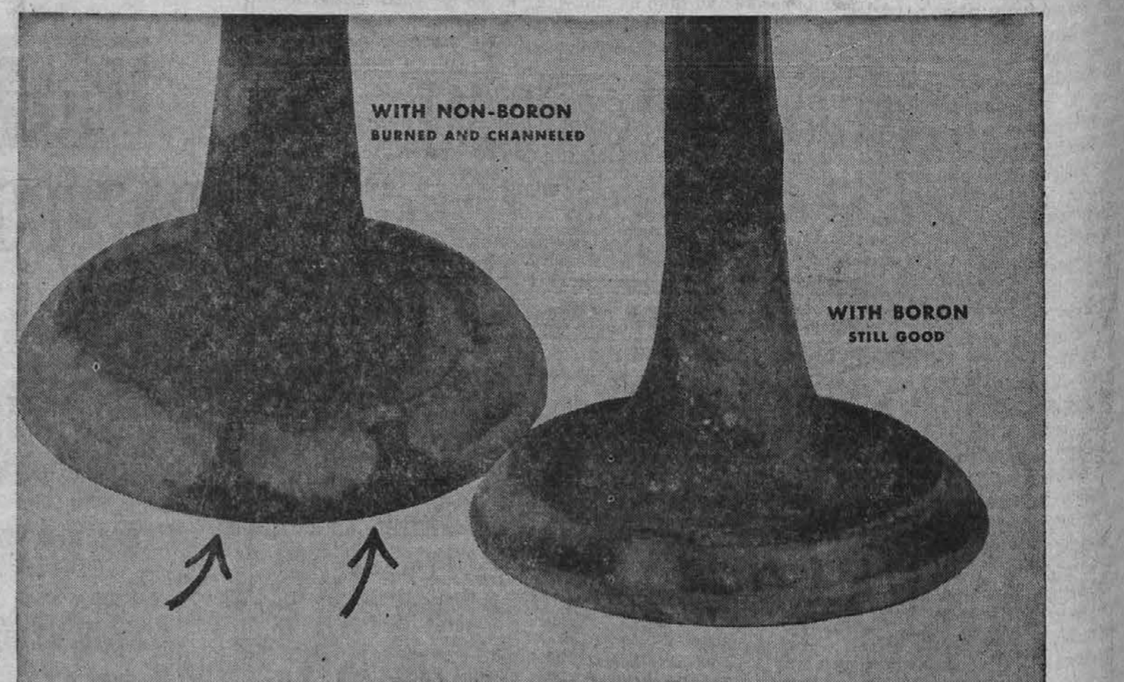
Te zaklopnici ste iz preizkusnih truckov, ki sta operirala pod enakimi okoliščinami. Zaklopka na levi, od trucka, ki ne rabi Boron gazolin, je opešala radi pretežkih vsedlin in zgorelih vrezov v zaklopki. Zaklopka na desni, iz trucka, ki rabi Boron gazolin, ima veliko manj vsedlin, lahko obratuje še za več tisoč milj.
