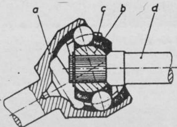
Fiksni homokinetični zglob a) čep, b) pesto, c) kletka, d) gred
