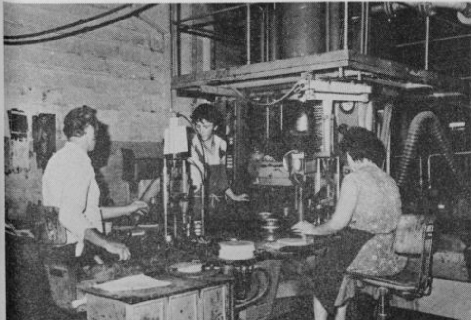
Proizvodnja visokoturažnih brusov v bakelitnem vezivu dosega visoko produktivnost že na klasičnih hidravličnih stiskalnicah, ki pa so v Cometovih delavnicah preurejene za tovrstno proizvodnjo ter do precejšnje stopnje mehanizirane in avtomatizirane.
