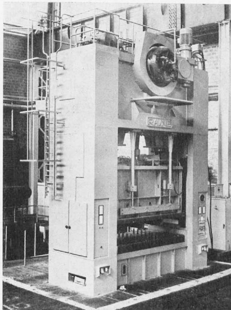
Za Gorenje — dvo- stebrna ekscentrična stiskalnica DQ 500
