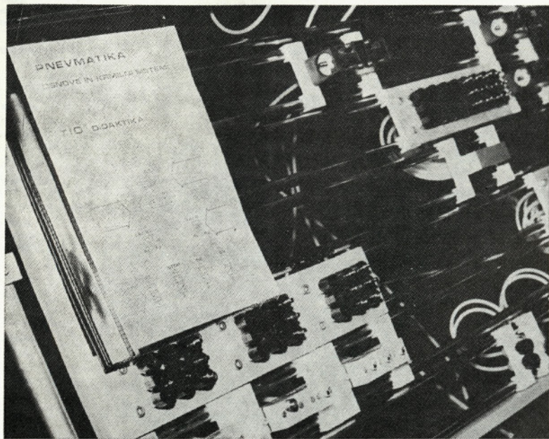
Delovni okvir na mizi Komplet z elementi in gradivom za pouk
