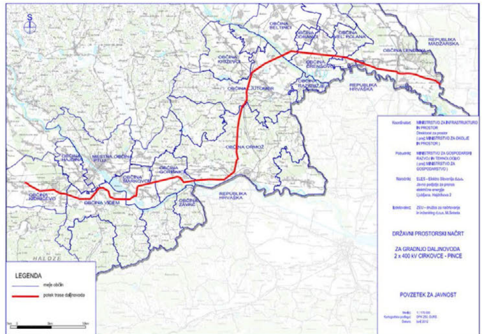
Skica daljnovoda
