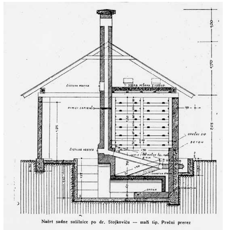
Načrt sadne sušilnice po dr. Stojkoviću, mali tip. Prečni prerez.
