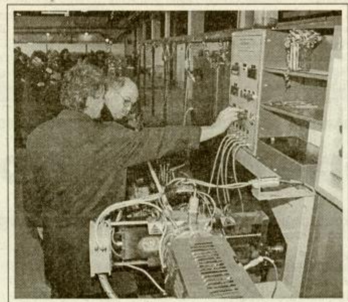
Jože Stanič je ob pomoči enega izmed delavcev pognal novo proizvodno linijo magnetnih tesnil za belo tehniko v podjetju Blues.
