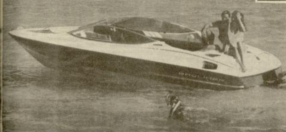
Motorni čoln Bayliner doseže hitrost 64 km/h. Dolg je 5,44 m, širok 2,13 m, njegova teža brez prikolice pa je 848 kg. Ima tudi zlozljivo streho in vgrajen stereo radiokasetofon.
