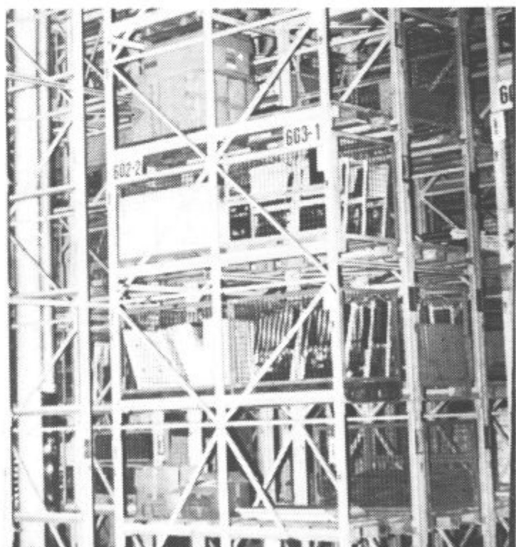
Visokoregalno skladišče za Servis TGO Gorenje Velenje
