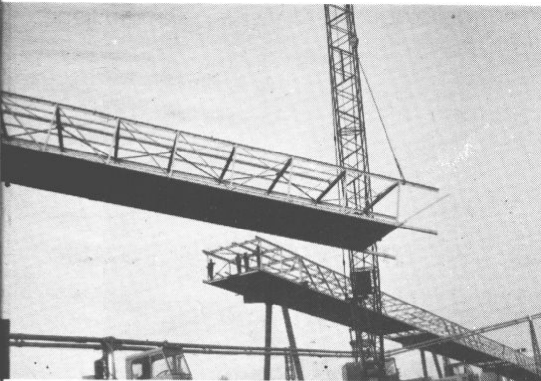
Mostovi za transport premoza za novo Termoelektrarno Šoštanj 4
