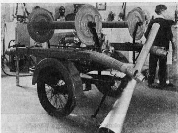
Z gasilske razstave: moderno in praktično orodje.
