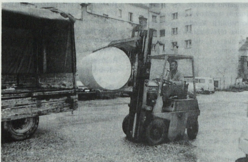
Delo z viličarjem — kleščarjem je lažje in varnejše — PAKO
