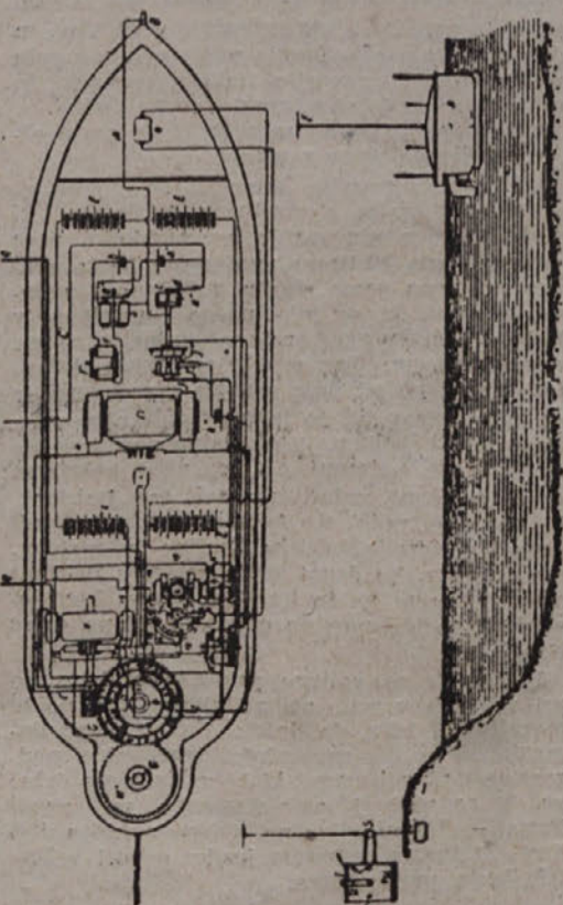
Original Teslinega patenta št. 613.809 z dne 1. julija 1898. Na sliki se vidi radijska oddajna postaja na obali in čoln z akumulatorsko baterijo, motorji in aparati za pogon ladje s pomočjo radijskih valov.
