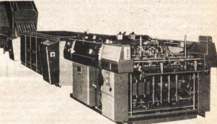
Sušilni kanal z elektronskimi nastavitvami, ki so ga izdelali strokovnjaki Etikete in priključili na italijanski tiskarski stroj, s čimer so dosegli večjo funkcionalnost stroja in kakovost.
