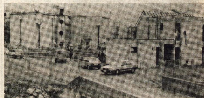
Nova mestna čistilna naprava na Jesenicah ima zmogljivost 30.000 ekvivalentov ali za 30.000 prebivalcev. Nanjo se bodo uporabniki priključevali postopoma, tudi s Hrušice in s Koroške Bele. Foto: F. Perdan
