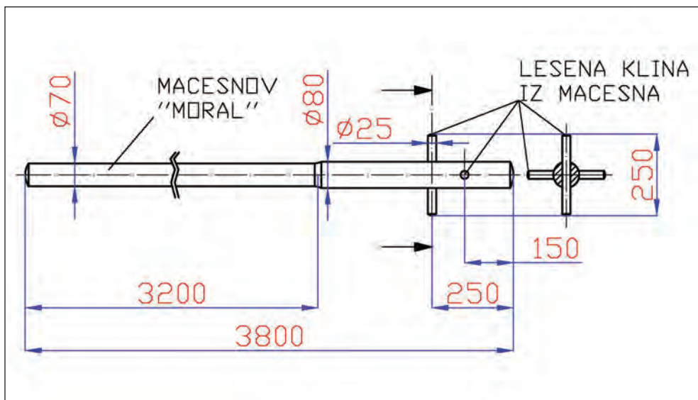
61. Načrt culegerja po navodilih (spominu) Toneta Rožmanca narisal njegov sin Simon Rožmanc avgusta 2017.
