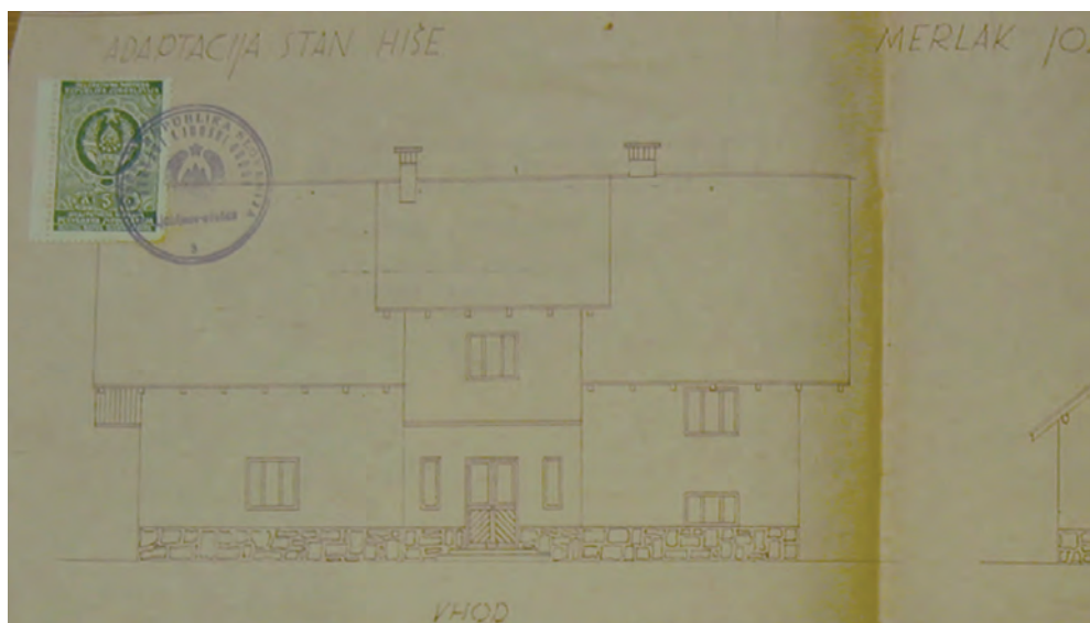
170. Načrt za prenovo hiše Jožeta Merlaka, pred letom 1954 (ZAL, VRH 10).
