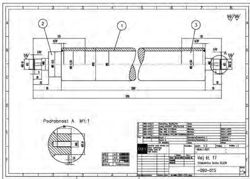
70. Načrt valja, del stiskalnice blata Klein. L. 2002 narisal in hrani Marko Garafolj.
