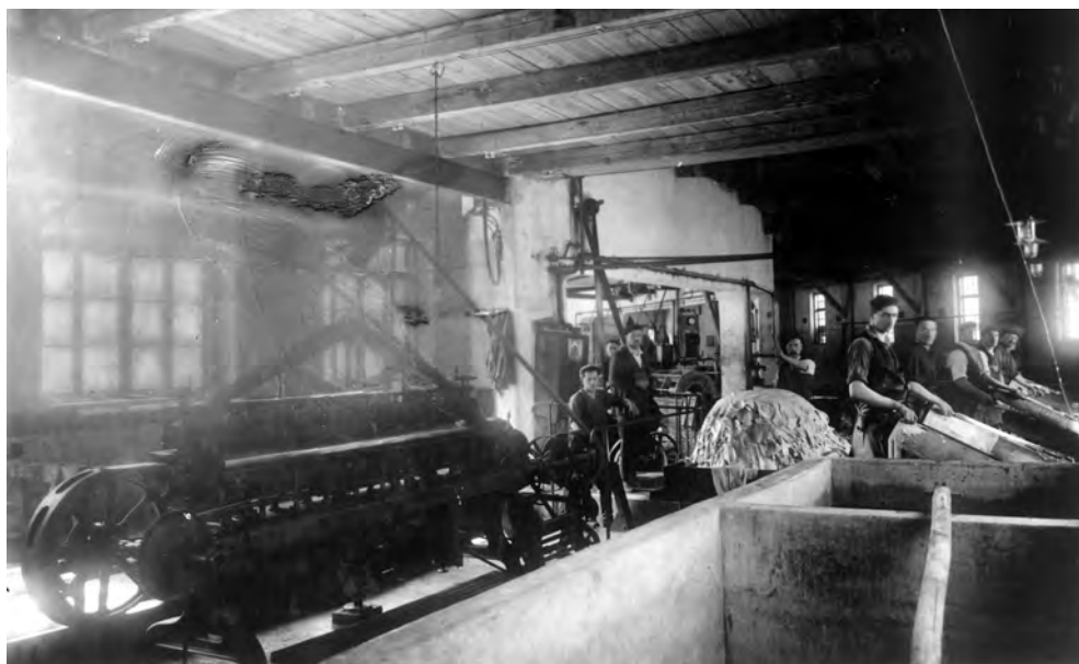
64. Notranjost Pollakove usnjarne na Vrhniki okrog leta 1930. Na levi Turnerjev cepilni stroj, desno lužilne jame s culegerjem , v ozadju usnjarji med delom. Avtor fotografije neznan. Muzejsko društvo Vrhnika.
