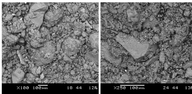
Slika 3.4: SEM mikroposnetek vzorca tufa (levo) in granulirane plavžne žindre (desno) Fig. 3.4: SEM of the tuff (left) and GGBS (right)
