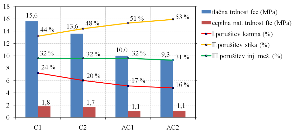
Slika 5.10: Povprečna tlačna in cepilna natezna trdnost valjastih preskušancev in zastopanost posameznih načinov porušitve pri cepilni natezni preiskavi
