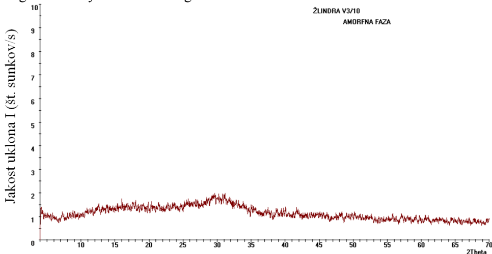
Slika 3.3: Difraktogram vzorca granulirane plavžne žlindre
