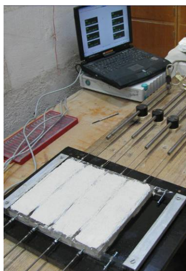
Slika 4.37: Povprečne deformacije malt M1 in M3a zaradi krčenja – prikaz postopka in rezultati Fig. 4.37: Average deformations due to shrinkage of mortars M1 and M3a – measurement procedure and results
