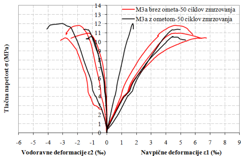
Slika 4.50: Rezultati tlačnih preiskav zidkov, sezidanih iz malte M3a brez ometa, in zidkov iz malte M3a z ometom, podvrženih 50-im ciklom zmrzovanja/tajanja
