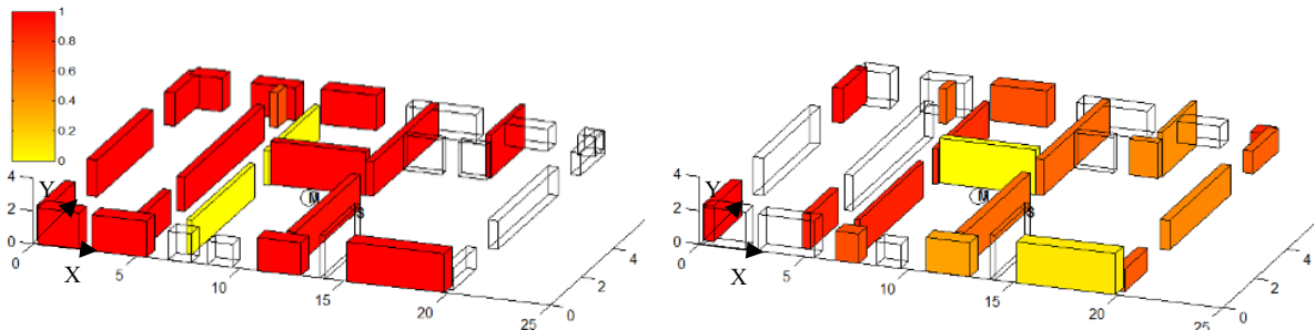
Slika 6.21: Izkoriščenost nosilnosti H_i/H_u (levo) in duktilnosti d/d_u (desno) za obstoječe – neinjektirano stanje pri MSN v smeri X
