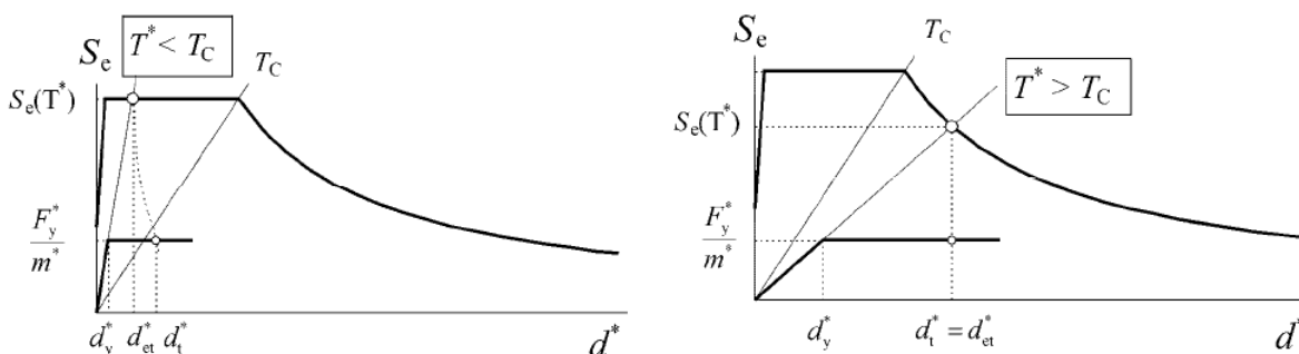
Slika 6.15: Določitev mejnega pomika za SDOF sistem v območju kratkih (levo) ter srednjih in dolgih nihanjnih časov (desno) Fig. 6.15: Determination of limit displacement for SDOF system in the range of short (left) and medium and long periods (right)
