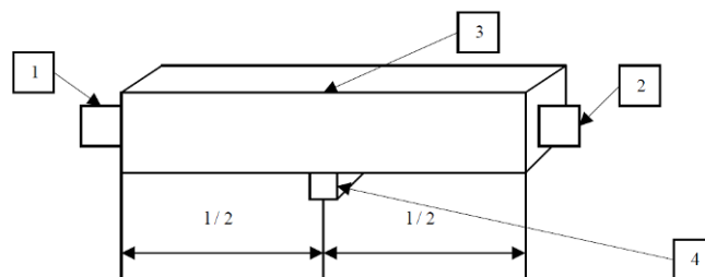
Slika 4.28: Postavitev pretvornikov za longitudinalno nihanje pri meritvah osnovne resonančne frekvence
