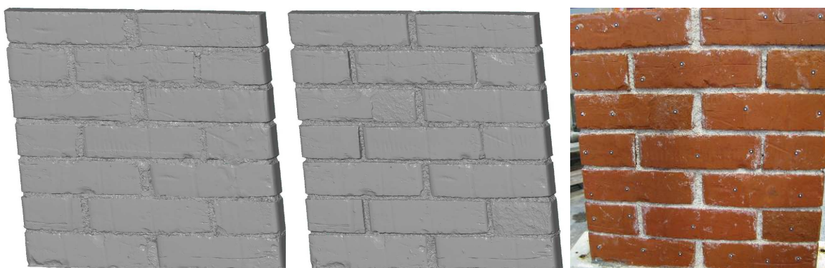
Slika 4.16: Iz leve: 3D model zidka M3a-6 pred ter 3D model in digitalni posnetek po 150-ih ciklih zmrzovanja/tanja
