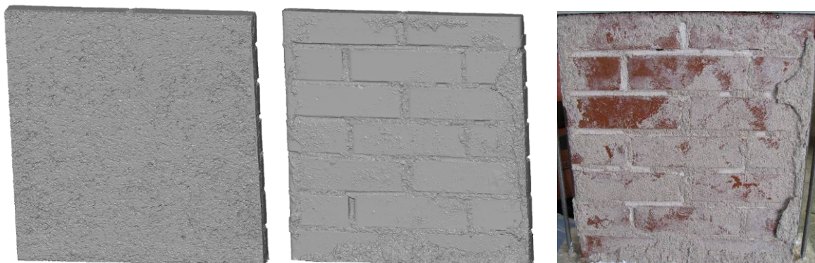
Slika 4.13: Iz leve: 3D model zidka M1-6 pred ter 3D model in digitalni posnetek po 50-ih ciklih zmrzovanja/tanja
