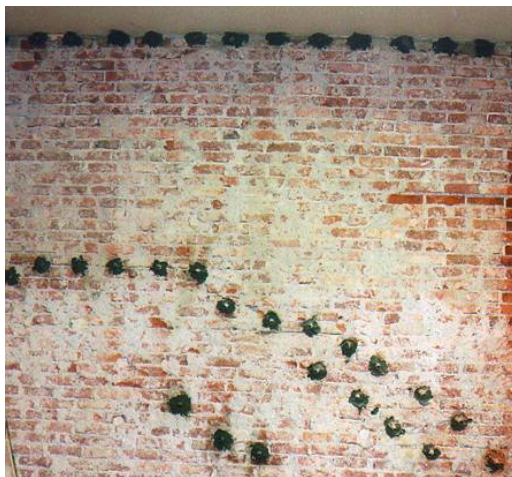
Slika 2.28: V zid vgrajeni nastavki pripravljeni za izvedbo linijskega injektiranja razpok Fig. 2.28: Set up of injection pipes for injection of cracks in brick masonry wall
