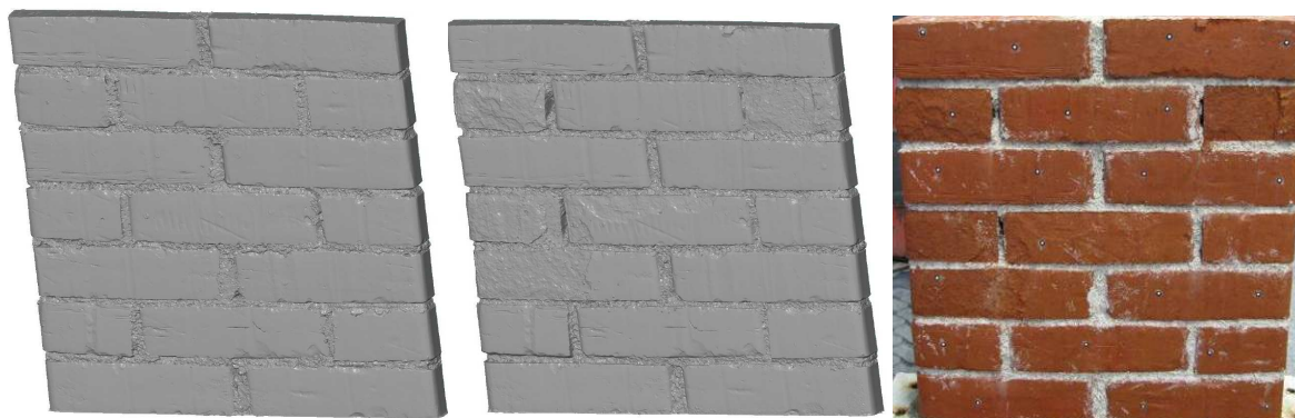
Slika 4.15: Iz leve: 3D model zidka M1-5 pred ter 3D model in digitalni posnetek po 150-ih ciklih zmrzovanja/tanja
