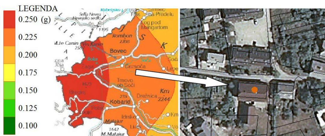
Slika 6.8: Izsek severo-zahodnega dela Slovenije iz karte potresne nevarnosti s prikazom lokacije objekta Čezsoča 76
