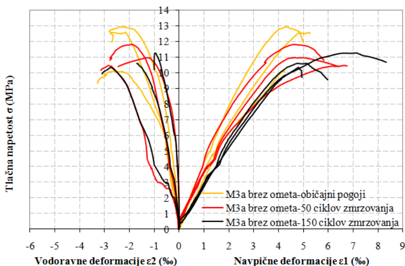
Slika 4.51: Rezultati tlačnih preiskav zidkov sezidanih iz malte M3a brez ometa pri običajnih pogojih nege ter po 50–ih in 150–ih ciklih zmrzovanja/tanja Fig. 4.51: Results of the compressive tests of the wallets M3a without plaster cured in normal conditions and after 50 and 150 freeze/thaw cycles
