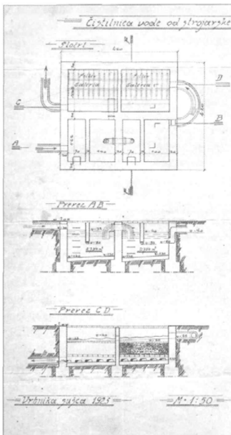
90. Načrt čistilne naprave strojarške delavnice Mihaela Tomšiča, 1904. (ZAL; VRH 2)
