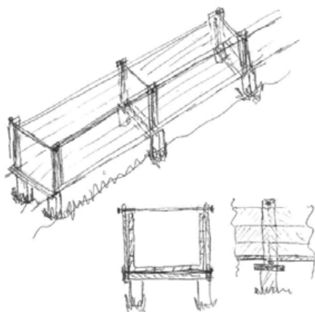
111. Leseno korito za vodo (Narisal prof. dr. B. Stanovnik) Leseno korito so nosili hrastovi stebri, ki so bili v parih zabiti v zemljo na razdalji 1 m ter 3 m oddaljeni od sosednjega para. Na vsak par stebrov je bila 50 cm nad tlemi položena prečna lega. Nanje so bili pritrjeni plohi, ki so tvorili dno korita. Stranice so bile prav tako iz plohov, pritrjenih na lesene opornice. Korito so spodaj in zgoraj povezale kovinske vezi, prвите z maticami.
