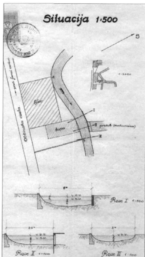
12. Situacija Stržinarjevega hleva in lope, 1904. (ZAL, VRH 2)
