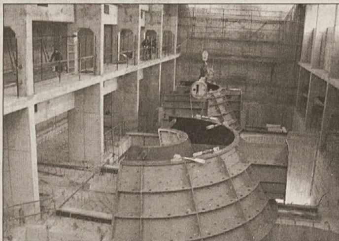
Spuščanje predvodilnika na temelje v strojnici
