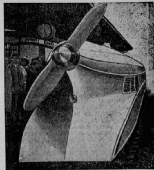
Progovni Zeppelin, voz s propelerjem, ki ga je zamislil in izvršil inž. Kruckenberg. Voz teče po tračnicah. Na poizkusni vožnji je zmagal prog Hamburg—Berlin, ki je 257 km dolga, v 1 uri in 38 minutah mestoma je doseglo vozilo brzino 230 km na uro.
