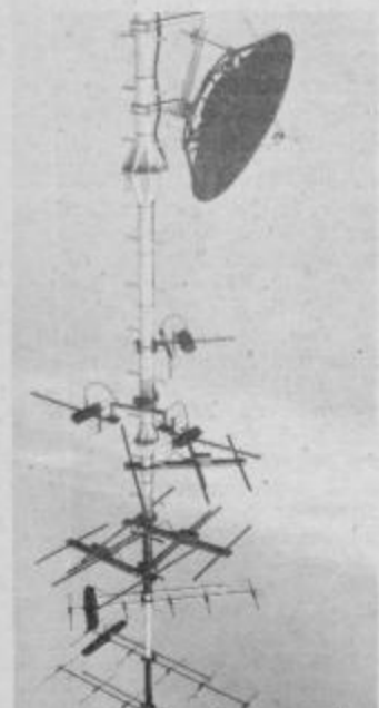
Sprejemni antenski sistem kableske televizije (CATV)
