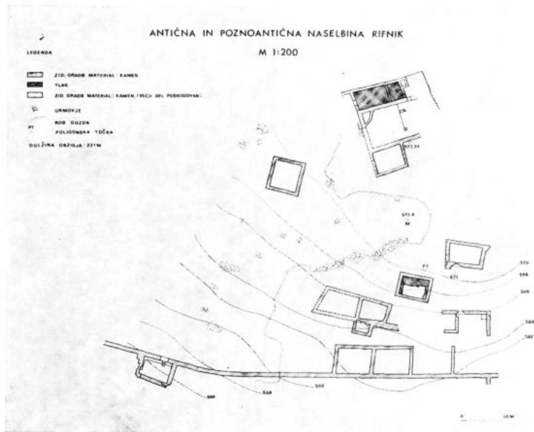
Sl. 2. Načrt poznoantične naselbine ob zaključku izkopavanj leta 1971. Vidna je stražarnica, dve na novo odkriti hiši in delno odkriti baziliki
