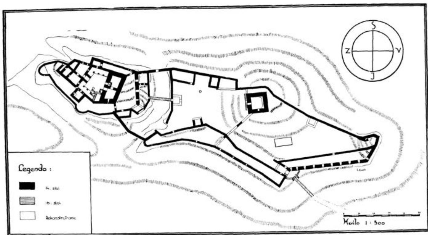
Sl. 41. Jože Turk: Grajski tloris (1957)
