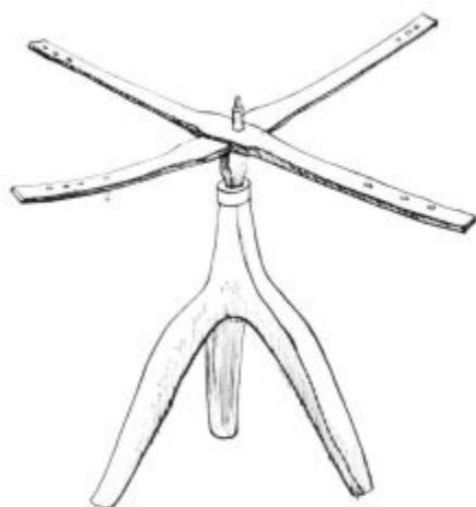
Motovilo za navijanje prediva (Oboje narisal Peter Krivec)
