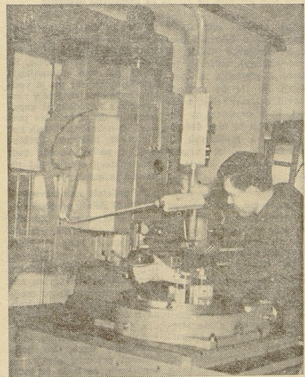
Jože Golob pripravlja precizni koordinatni vrtni stroj za prve naloge v naši novi orodjarni
