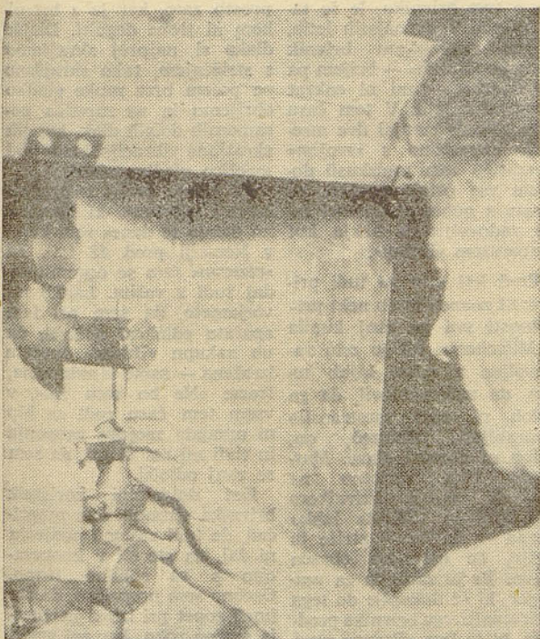
Iz obrata tovarne električnih aparatov v Dobrepolju: Anton Novak pri punktiranju (električnem varjenju) sestavnih delov RB-2
