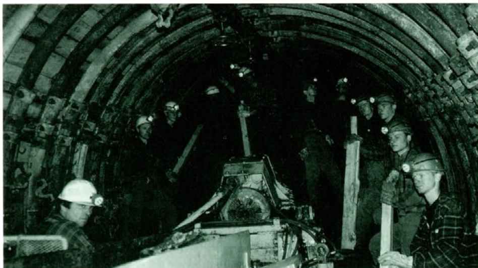
Praktični pouk dijakov pri strojni izdelavi jamskih prostorov na pripravi številka 1 in zalaganju stropnega loka. Na fotografiji so inštruktor Drago Zrnič in dijaki na desni ter moštvo priprav na levi strani.
