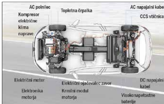
Pogonski sklop električnega VW golfa (foto: Avtofokus)
