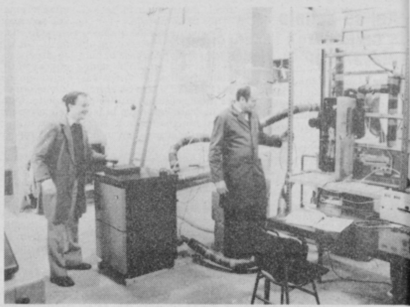
Jože Kaplar iz Strojne fakultete in Lojze Rak iz Gradnje pri merjenju v novem laboratoriju. Preizkus enega kotla traja neprekinjeno 36 ur, pri tem pa spremljajo štiriindvajsetih merilnih mest.
