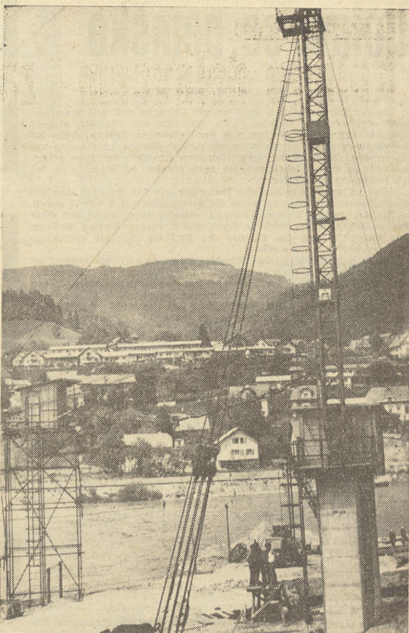
ZGORAJ: Novi most v Dravogradu bo dolg 216 metrov in bo grajen v železobetonski konstrukciji s prednapetimi nosilci
