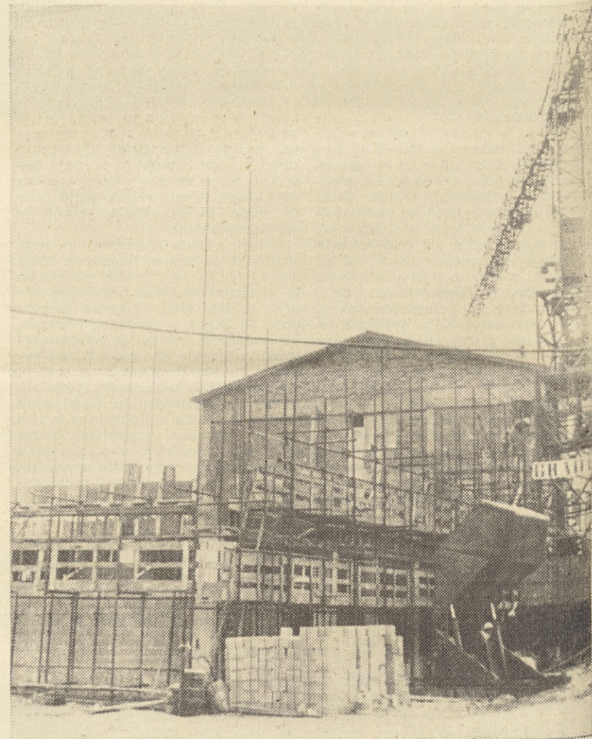
Ob pričetku del na novem gradbišču Aero v Celju
