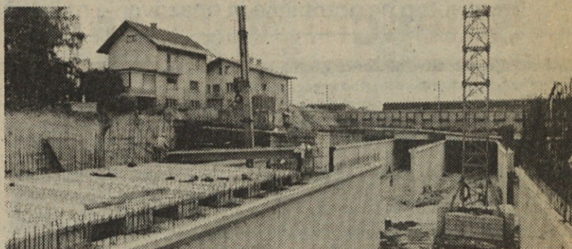
Montaža nosilcev na prvem delu šentviške »galerije« gre že h koncu
