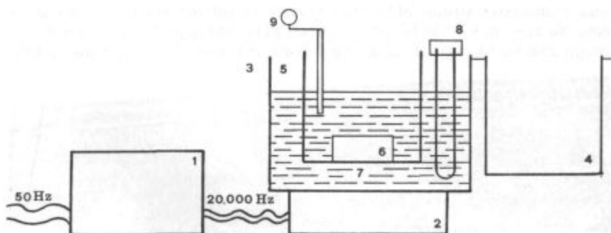
Sl. 10. Shema delovanja ultrazvočne aparature
