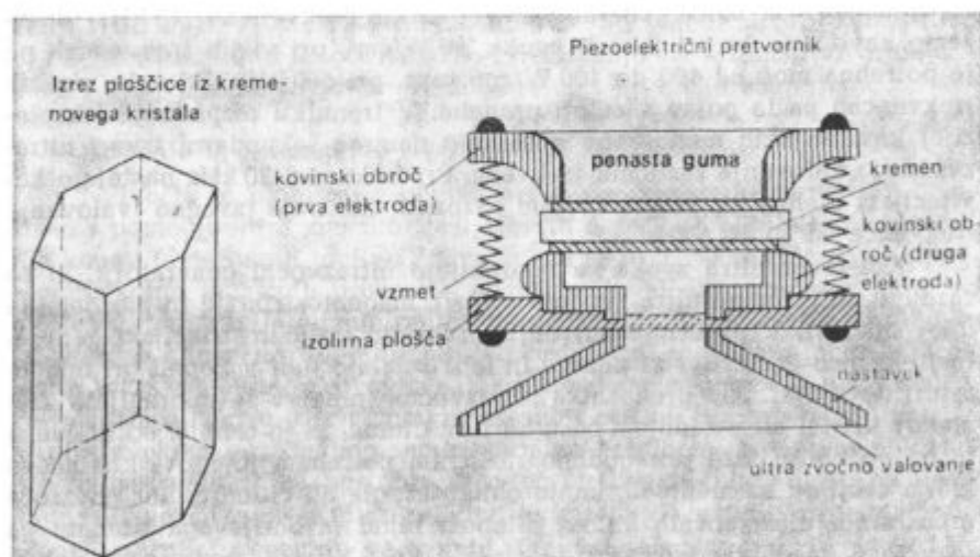
Sl. 9. Ultrazvočni pretvorniki
