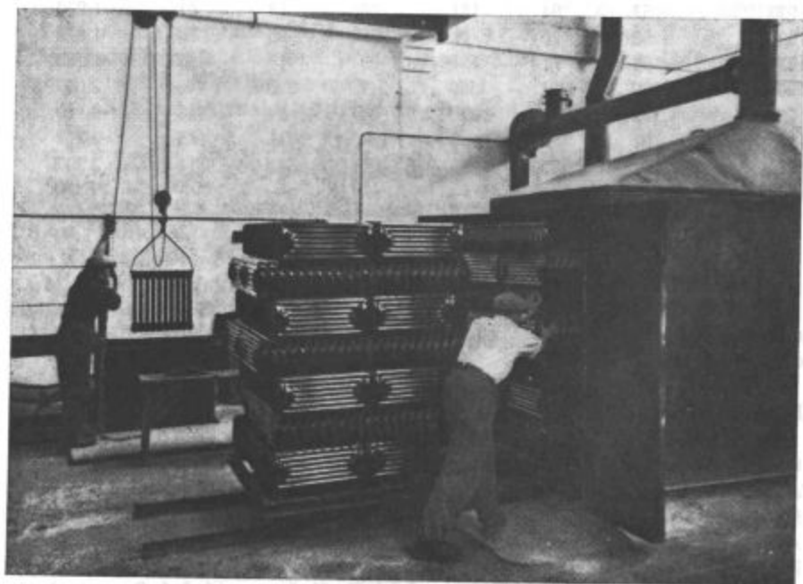
Prva sušilna peč za radiatorje (1932)
