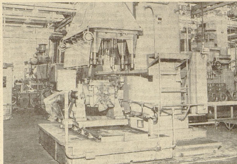
Linija za obdelavo ohišja transmisije
